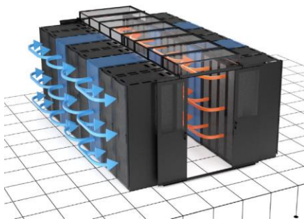
Системы изоляции «горячих» коридоров
